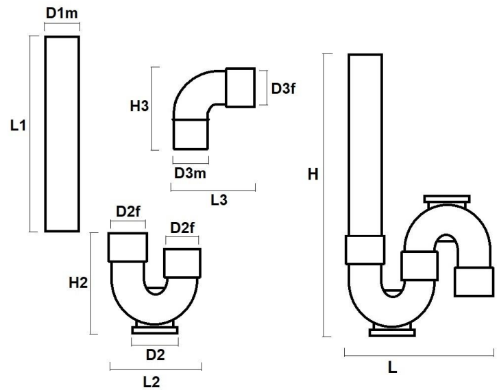
SMV40 Siphon de machine à laver sortie verticale
