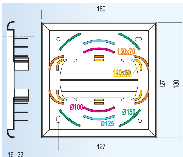
Grille "GU1818B" ABS en applique avec volets anti pluie
