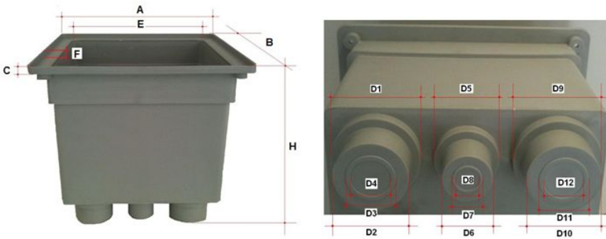
BOX DIMENSIONS
