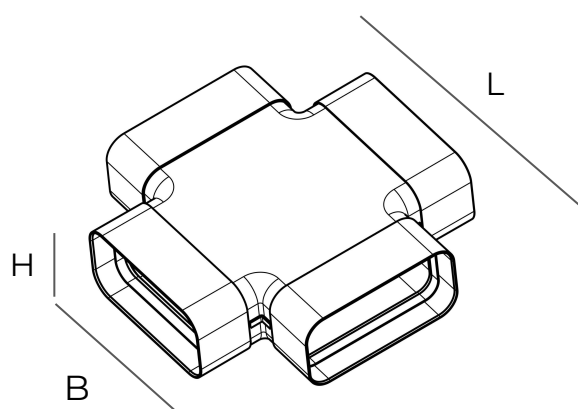
CRX157B Raccord plat ABS à 4 voies FFFF
